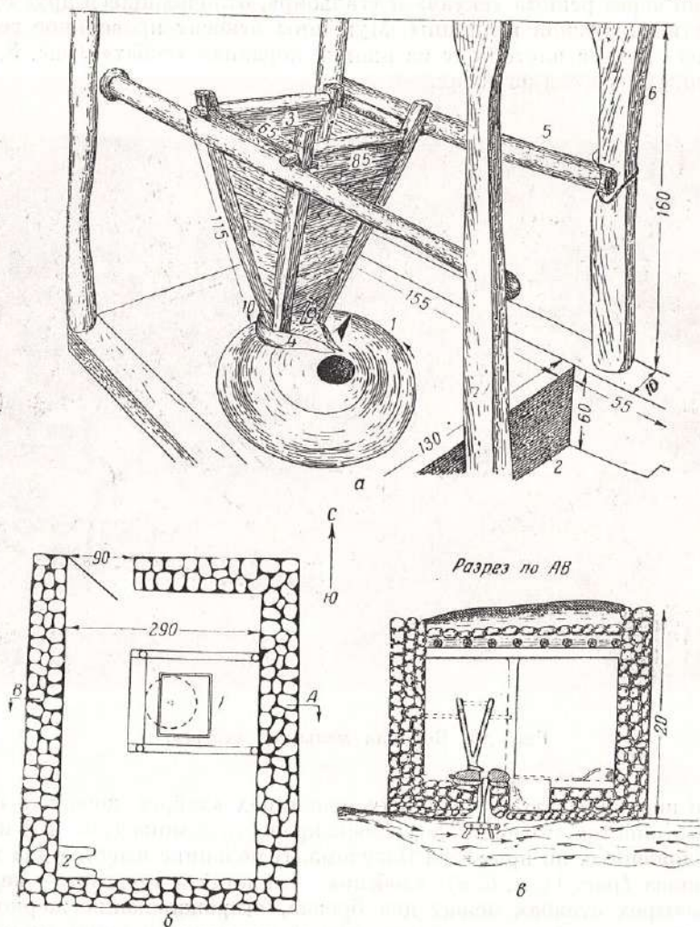
Рис. 11. Водяная мельница «хаэрг»:
