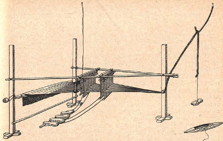
Рис. 8. Горизонтальный гапакский станок для изготовления шерстяных и хлопчатобумажных тканей, г. Хорог, Областной краеведческий музей (рис. Р. Разинчевой)
