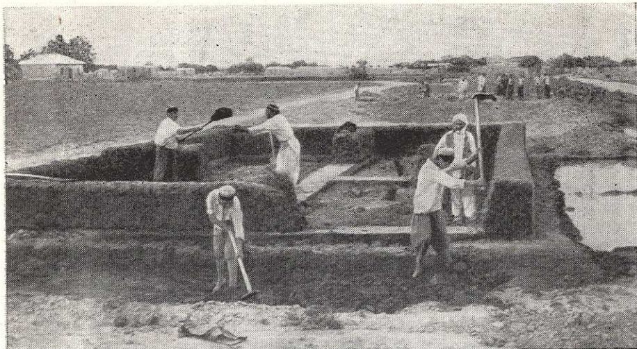
Возведение пахсовых стен дома (к. Сазган; фото Н. С. Кармазина)
