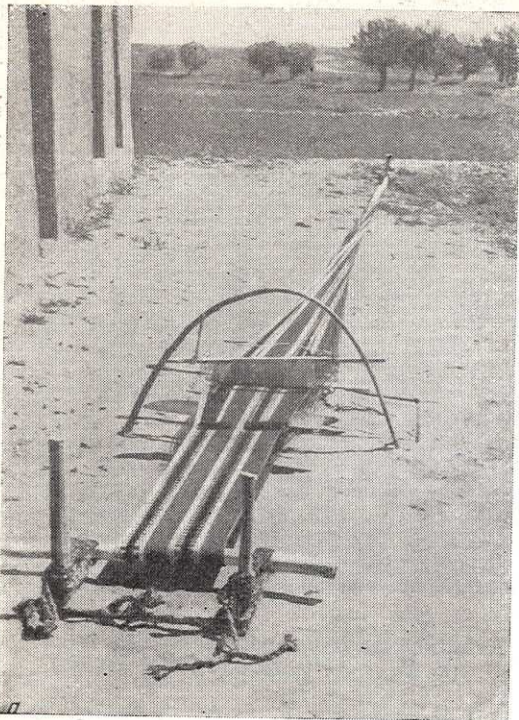
Ткацкий станок урмак (к. Сазаган; фото Н. С. Кармазина)
