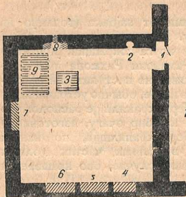
Рис. 15. Комната для гостей в доме Мирзо в сел. Номиткон. 1 — дверь в rešvōn; 2 — очаг; 3 — сандали; 4—7 ниши; 8 — окно в нише; 9 — место для гостей (шкура барана); 10 — rešvōn.
