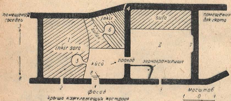
Рис. 19. Жилище Джума Одина в сел. Дехи-балайд. I — mür ; II — kánna ; 1 — дверь; 2—4 — окна; 5—6 — очаги; 7 — ниша; 8 — лестница из каменных плит.
