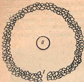
Рис. 30. План „дома для гостей“, летовка Куливорсоуг. 1—стена каменной кладки; 2—жерди; 3—слой щебня и земли; 4—балки; 5—отверстие для выхода дыма; I—проход; II—место для костра.
