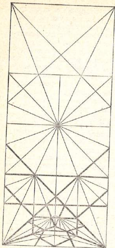
Декоративные своды в караван-сараяе.
