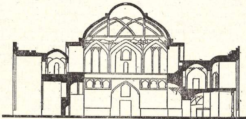
Купольные системы: а) Токи Саррофон, б) Токи Тильпакфурушон, в) Хонако Бахаведдин (XVI в.).
