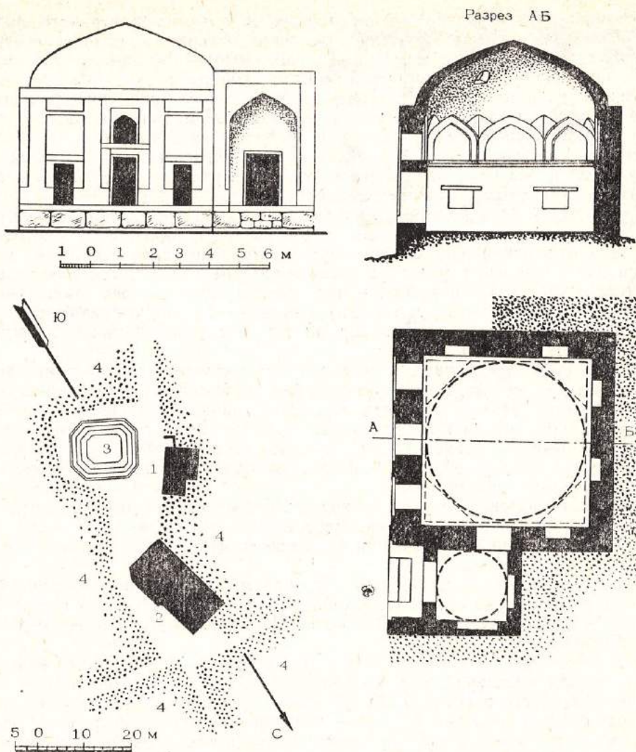
Мақтаб в гузаре Кози Файзи. План, фасад и разрез
