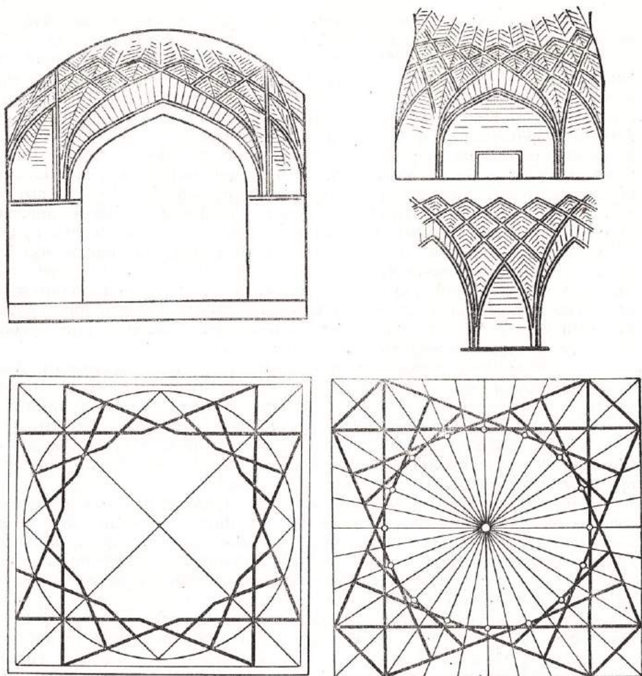
Шитовидные своды в медресе Кукалдош (XVI в.).
