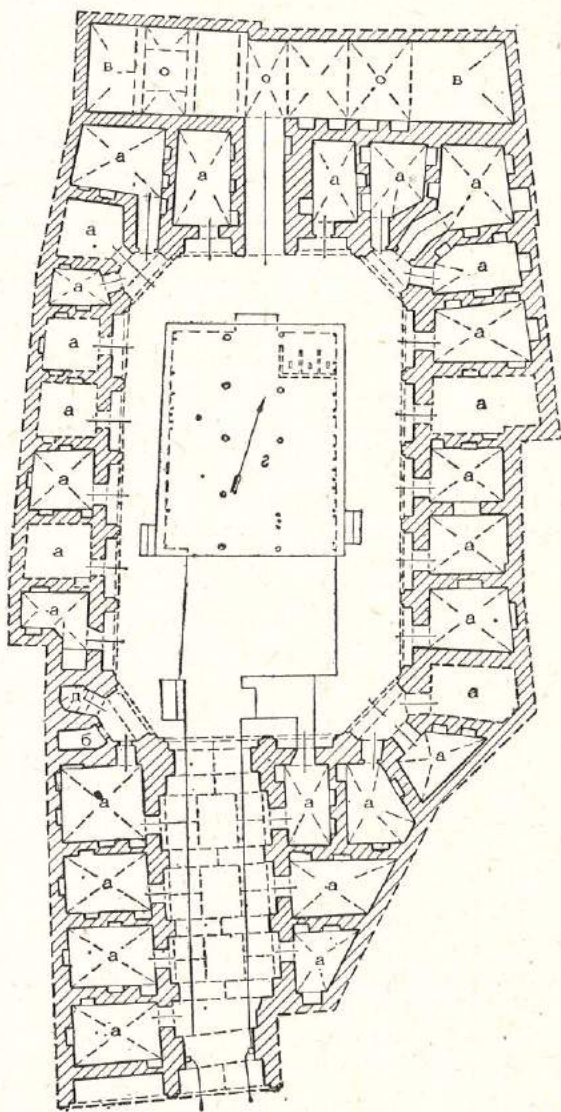
Караван-сарай Кулота. План.
