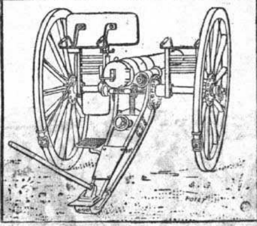
Скорострѣльная пушка Максима-Норденфельда на полевомъ лафетѣ.
