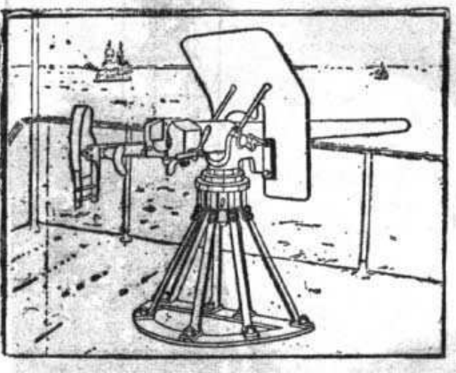
Скорострѣльная пушка Гочкиса, образца 1896 г.
