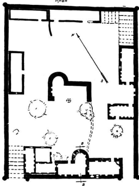
Рис. 52. Кувакский район. План ховлы Роушан Мерета и разрез по кумезу
