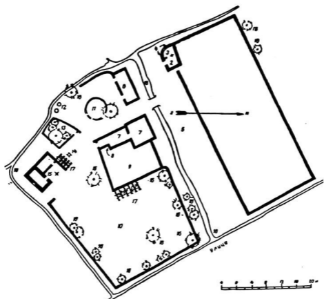
Рис. 49. Астана-Баба. Ховлы Джума Джабарова. План участка 1 — посевы пшеницы; 2 — открытый дворик; 3 — навес; 4 — продукты на уровне земли; 5 — проезд между приусадебными постройками; 6 — жилое зимнее помещение; 7 — склад топлива и хозяйственного инвентаря; 8 — окно-лаз; 9 — посев лука и моркови; 10 — посев джугары; 11 — летнее жилое помещение (юрта); 12 — очаг и тандыр; 13 — загон для скота; 14 — колодезь; 15 — жилое зимнее помещение с айваном и саманханой; 16 — древесные насаждения; 17 — виноградник; 18 — зрык
