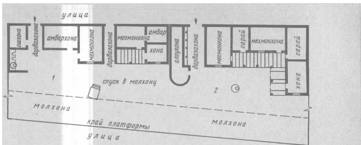
Рис. 2. Планы жилых домов: 1 — Ходжи Саидназарова, 2 — Ниезахмеда Ибрагимова
