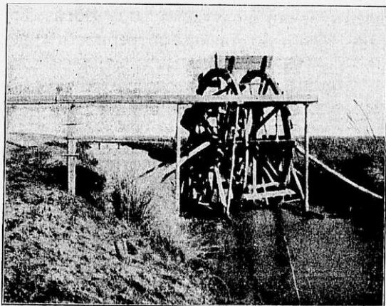
9. Водоподъемное колесо (чигирь). Образецъ недорогого примитивнаго сооруженія.
