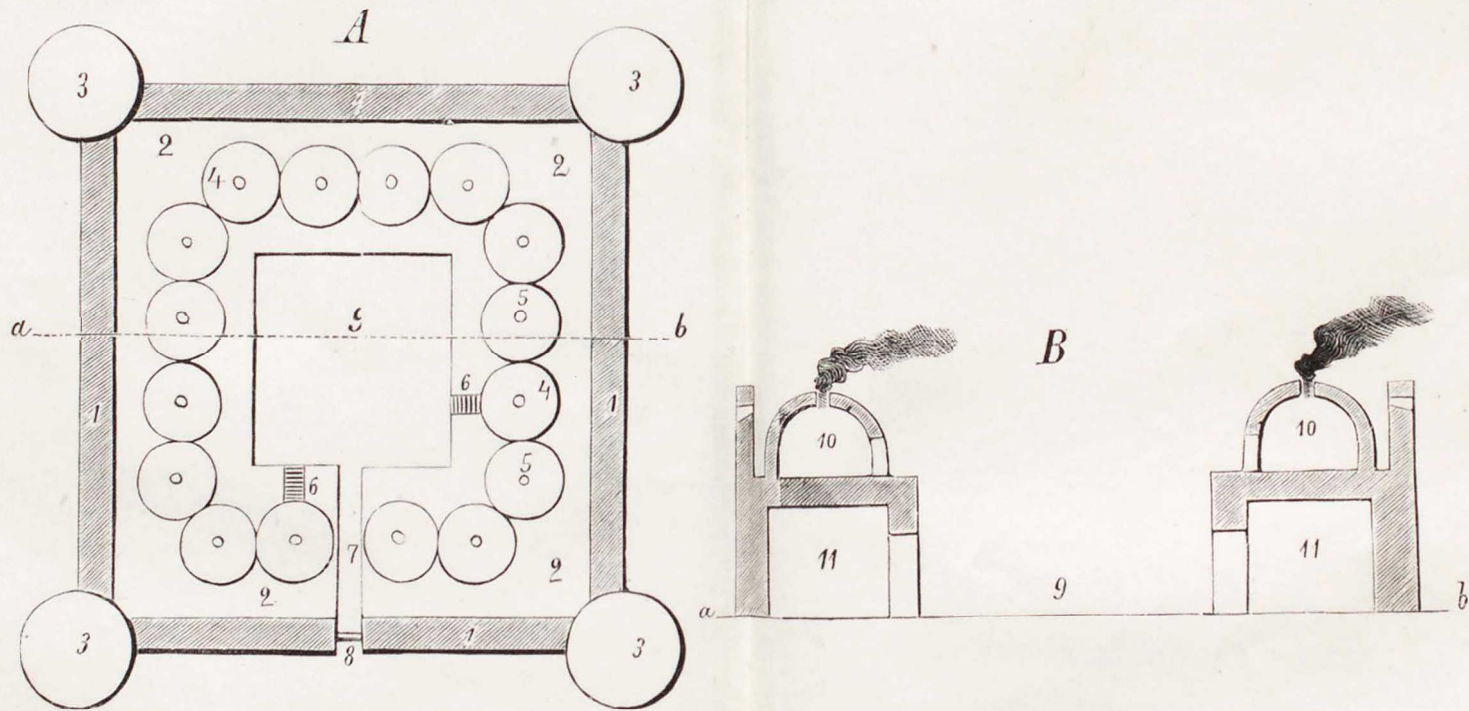
А. Планъ селенія Шормасъ; В. Профиль по линіи ab ; 1) наружная стѣна; 2) крыша нижняго этажа, на которой поставлены куполообразные жилые дома; 3) башня; 4) куполообразные жилые дома; 5) отверстія для дыма; 6) лѣстница; 7) проходъ; 8) ворота; 9) общій видъ; 10) жилой домъ; 11) нижній этажъ для скота.
