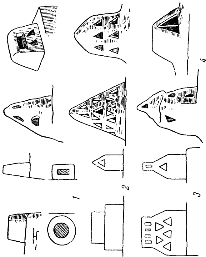
Рис. 8. Дымовые трубы: 1 и 2 — Захматабад; 3 — Сангистон; 4 — Вашан
