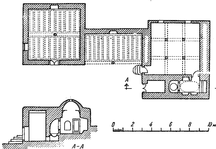
Рис. 14. Мечеть в Рарзе. План и разрез
