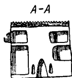
Рис. 9. Дом в Сарытаге. План и разрез худжры: I — хона; II — худжра; III — айван; IV — огул (помещение для овец); V — дарваза (крытые ворота); 1 — тахтахона; 2 — ташнаб; (водослив); 3 — оштон; 4 — кавш-каши, 5 — сым-каши
