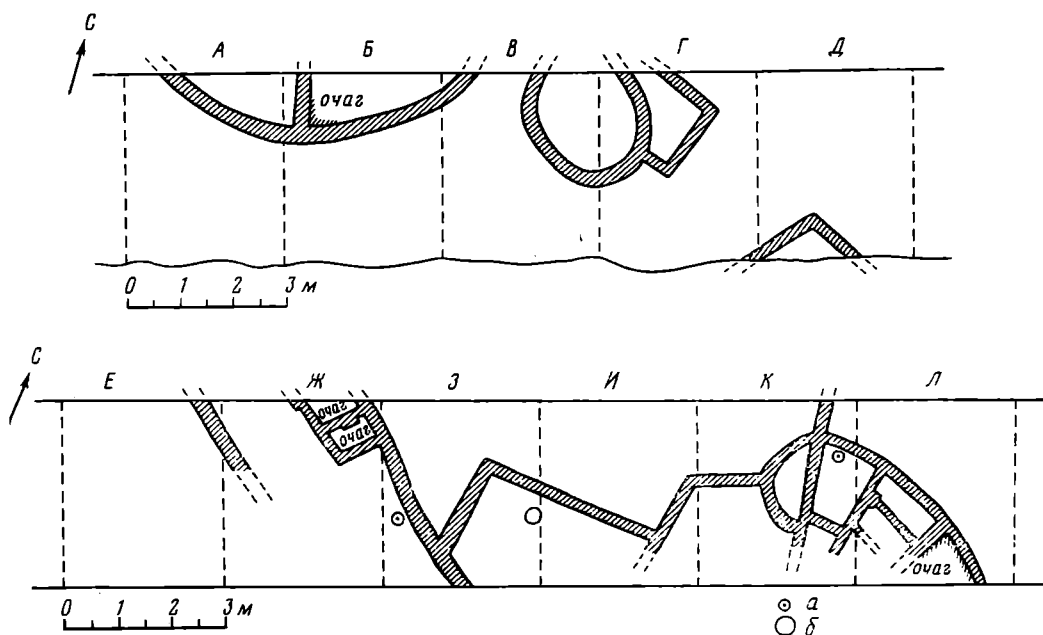
Рис. 2. А — строительные остатки строений слоя 4 северного холма Анау; Б — строительные остатки строений слоя 5 северного холма Анау; а — подпорок; б — вкопанная в пол корчага
