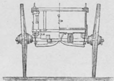
Аптечная двуколка, видъ сзади.
