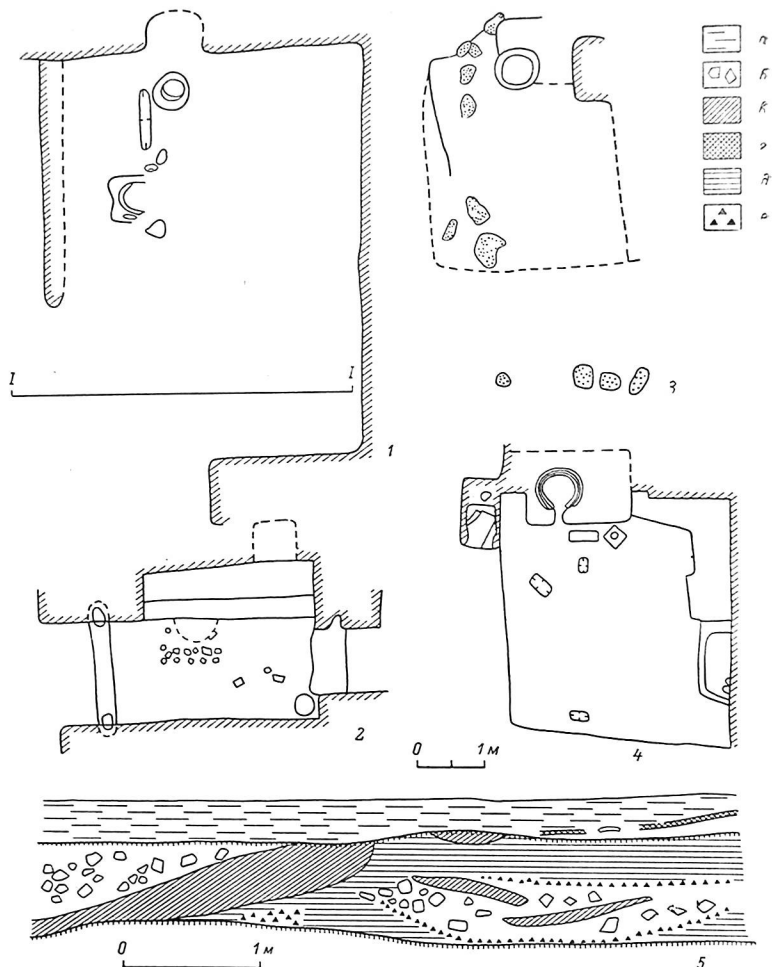
Рис. 7. Пемпдикент. Объект XVI. Планы металлообрабатывающих мастерских.
