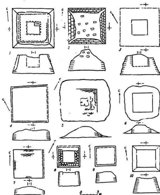
Рис. 75. Планы и разрезы башен Устьюрта:
