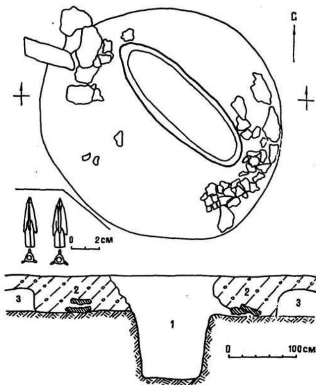
Рис. 54. Курганная группа Касажол. Кургan 6, план, разрез, находки: 1 — илочно-илуное заполнение ямы, 2 — каменное кольцо на горизонте, 3 — валик выкида. На врезке — наконечники стрел.
