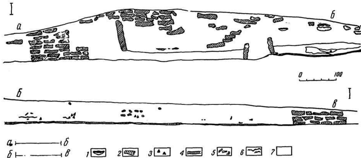
Рис. 63. Разрез I—I отдельной постройки Сумбетимералан—Куркреук. Условные обозначения:
