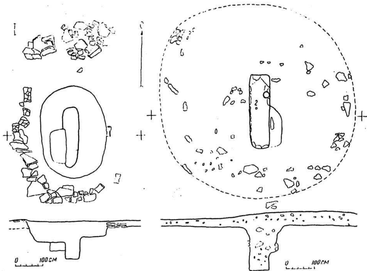
Рис. 57. Курганная группа Биркалпашиниграу-2; I — курган I, план и разрез; II — курган 2, план и разрез; 1 — сосуд, 2 — пряслице.
