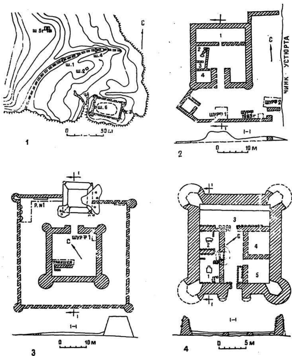
Рис. 68. Планы городищ Устьюрта:
