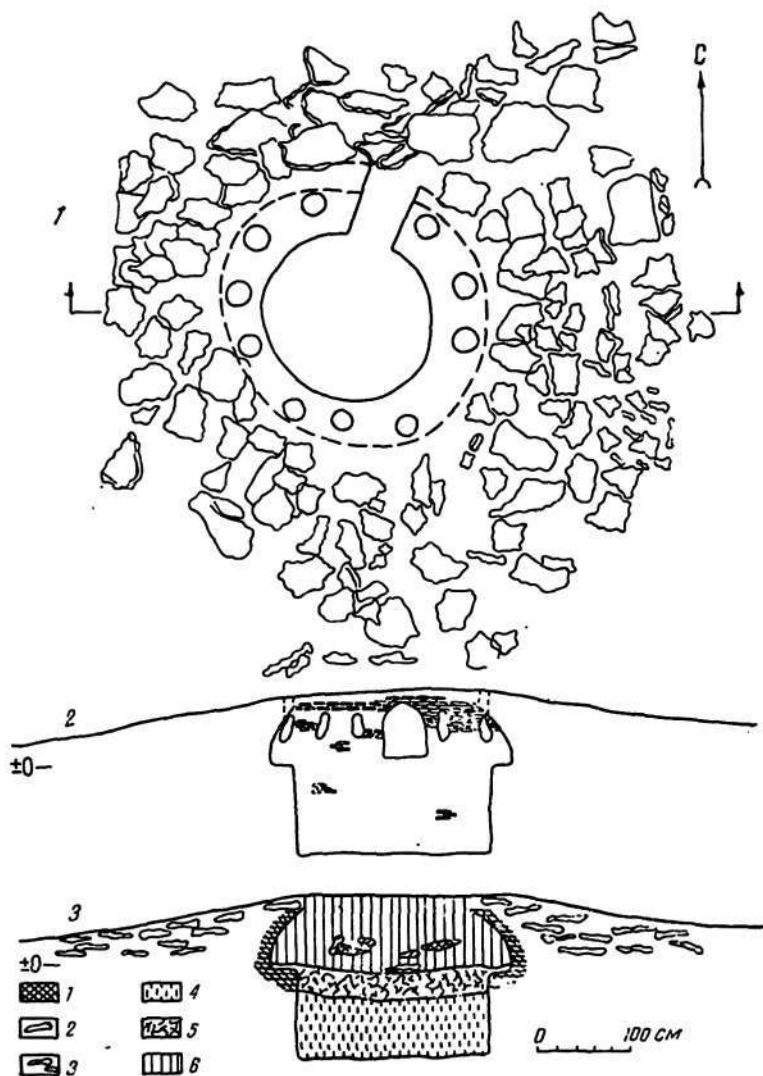
Рис. 85. Гончарная печь у городища Курганча, план и разрезы:
