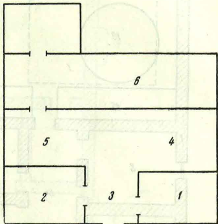
Рис. 6. Схематический план жилого туркменского дома начала XX в. (Аму-Дарьинский отдел, местность Шурахан). 1 — михман-хана; 2 — галяль-хана; 3, 4 — айван; 5 — сенс-хана; 6 — самап-хана.
