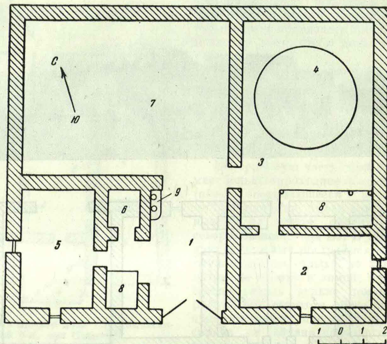
Рис. 4. План жилого дома (Калининский р-н Ташаузской обл.).
