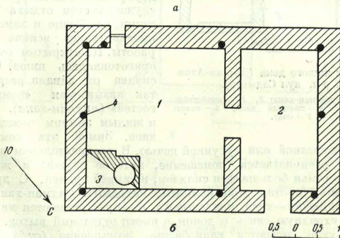
Рис. 1. «Там-кепше» — постройка старого типа (Дарган-Атинский р-н Чарджоуской обл. ТССР): а — общий вид; б — план.
