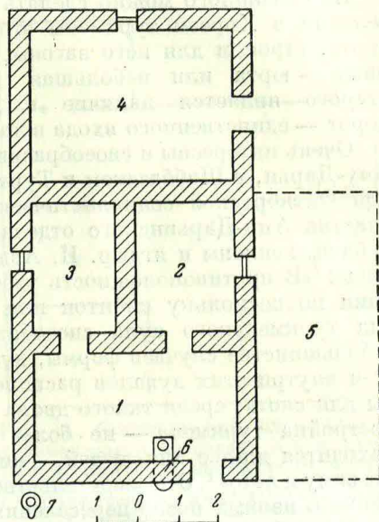
Рис. 5. План жилого дома (Калининский р-н Ташаузской обл.).
