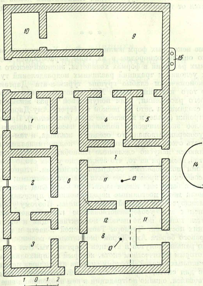
Рис. 8. План жилого дома (Турткульский р-н КК АССР).
