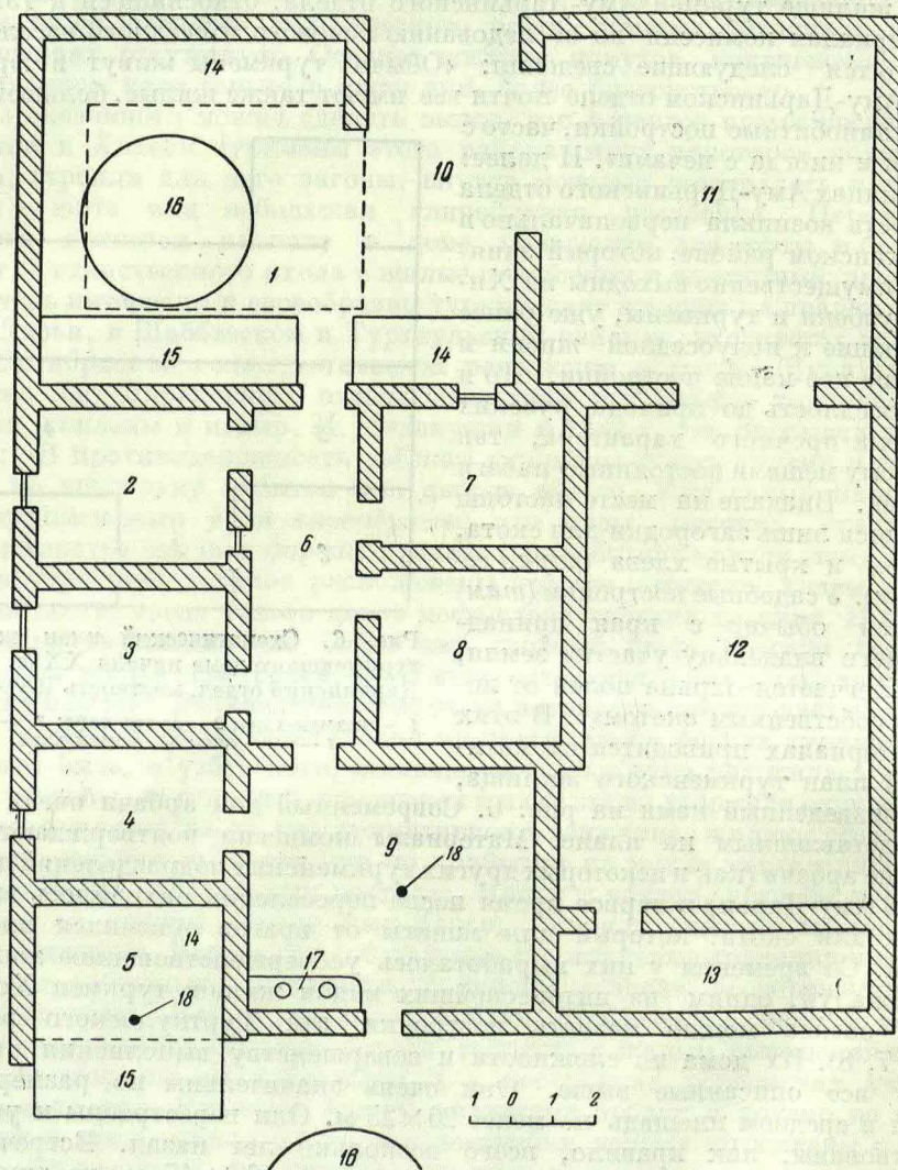
Рис. 7. План жилого дома (Турткульский р-н КК АССР).
