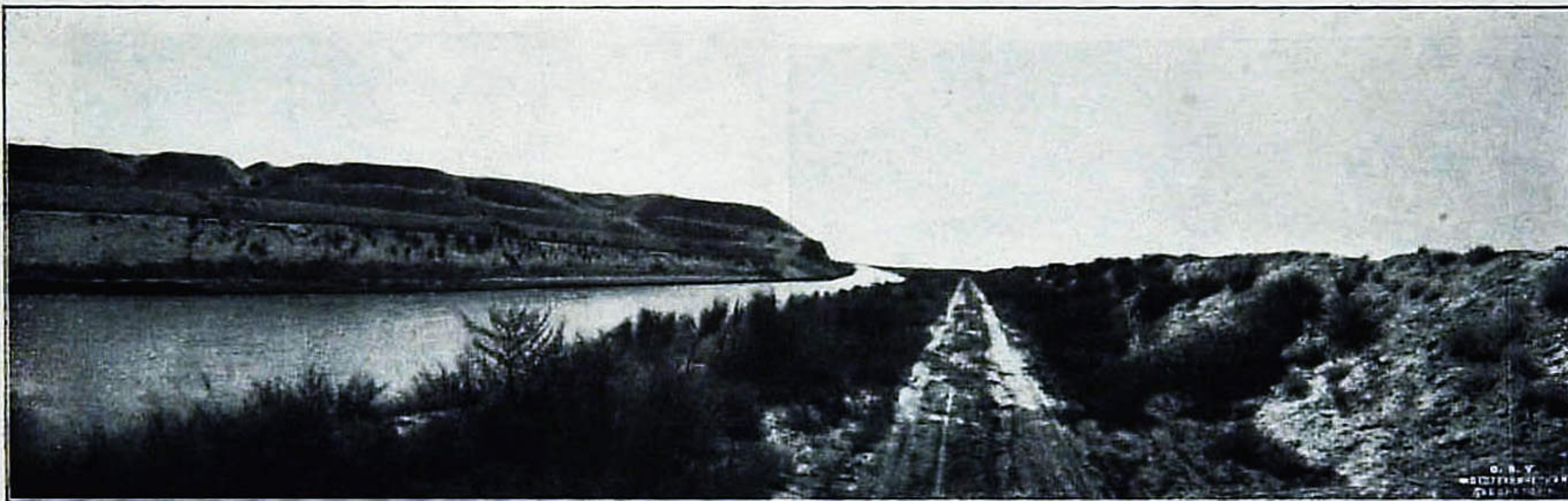
Видъ Романовскаго канала на 12 верстѣ, внизъ по теченію.
