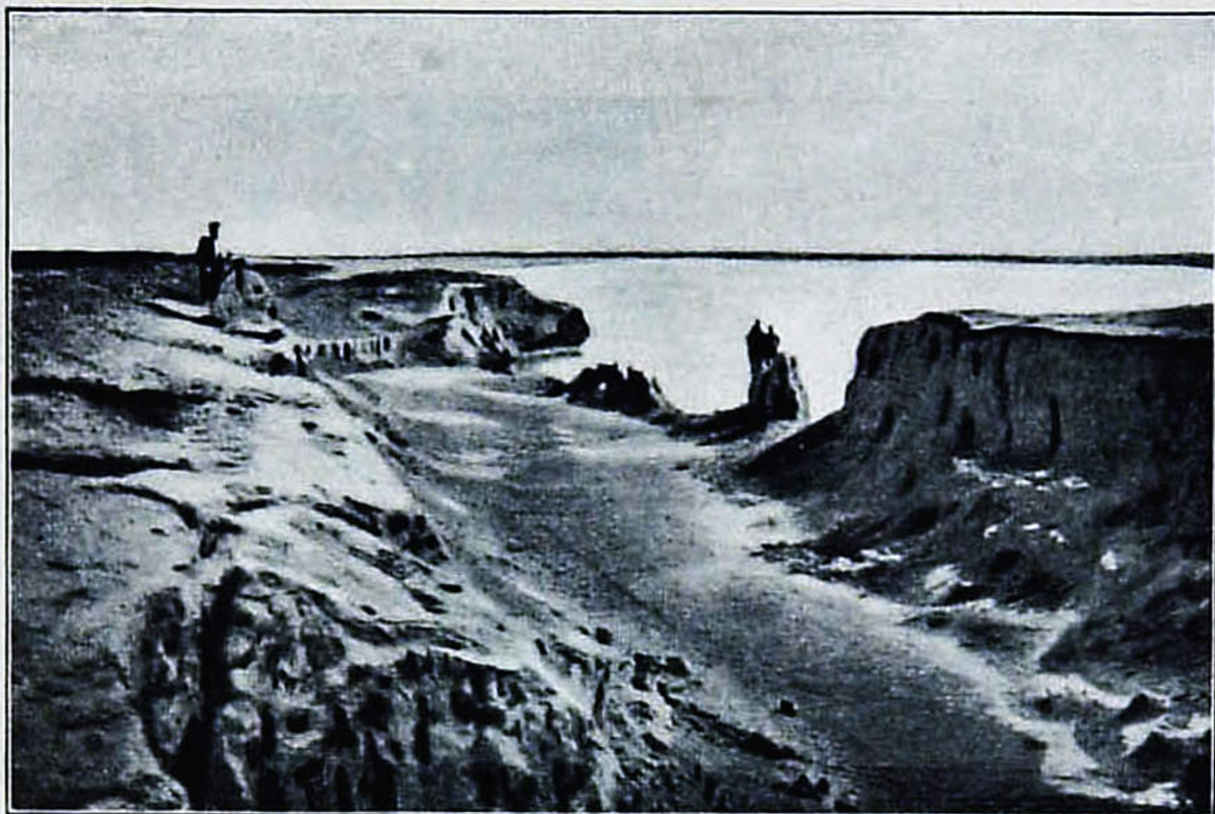
Размывъ канала Императора Николая I Сыръ-Дарьей на 30-й верстѣ, у озера Алка-куль въ 1910 г. Видъ внизъ по теченію.
