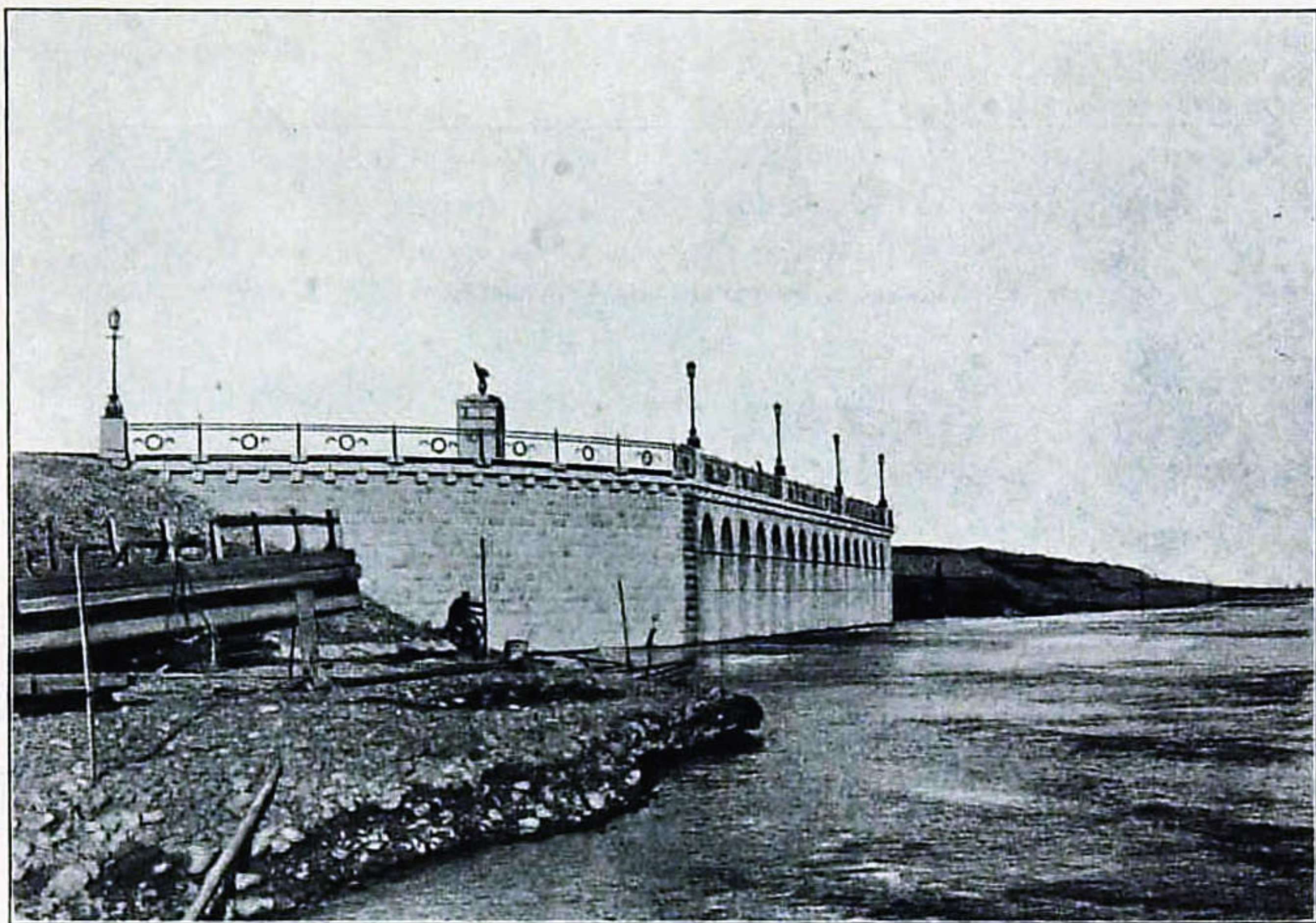
Головной шлюз Романовского канала со стороны р. Сырь-Дарьи.
