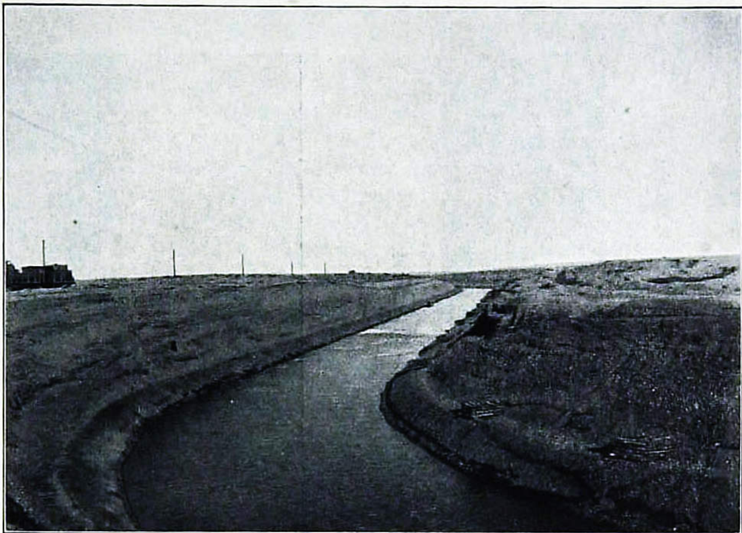
Первая верста Романовского канала.
