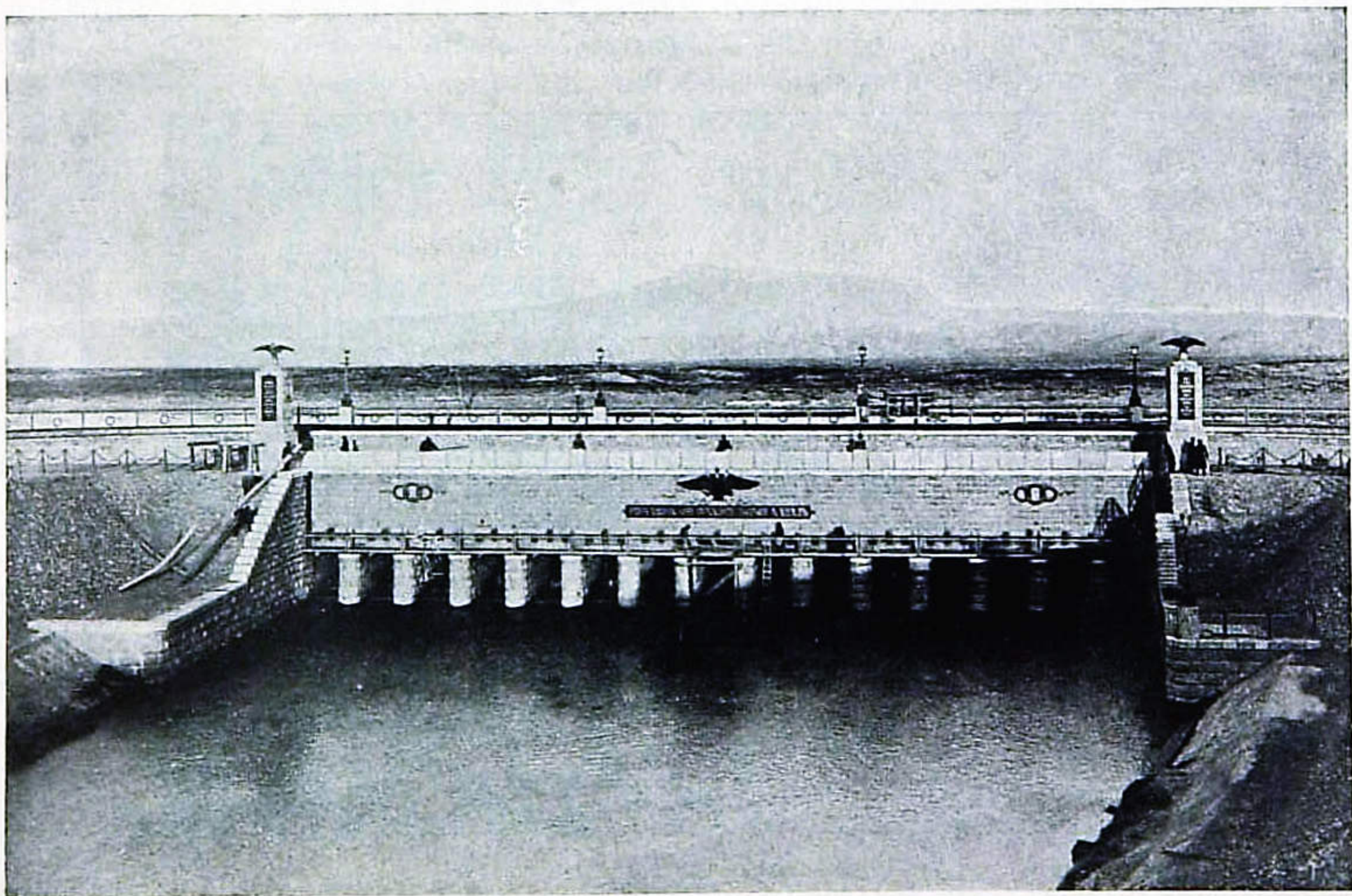
Головной шлюз Романовского оросительного канала.
