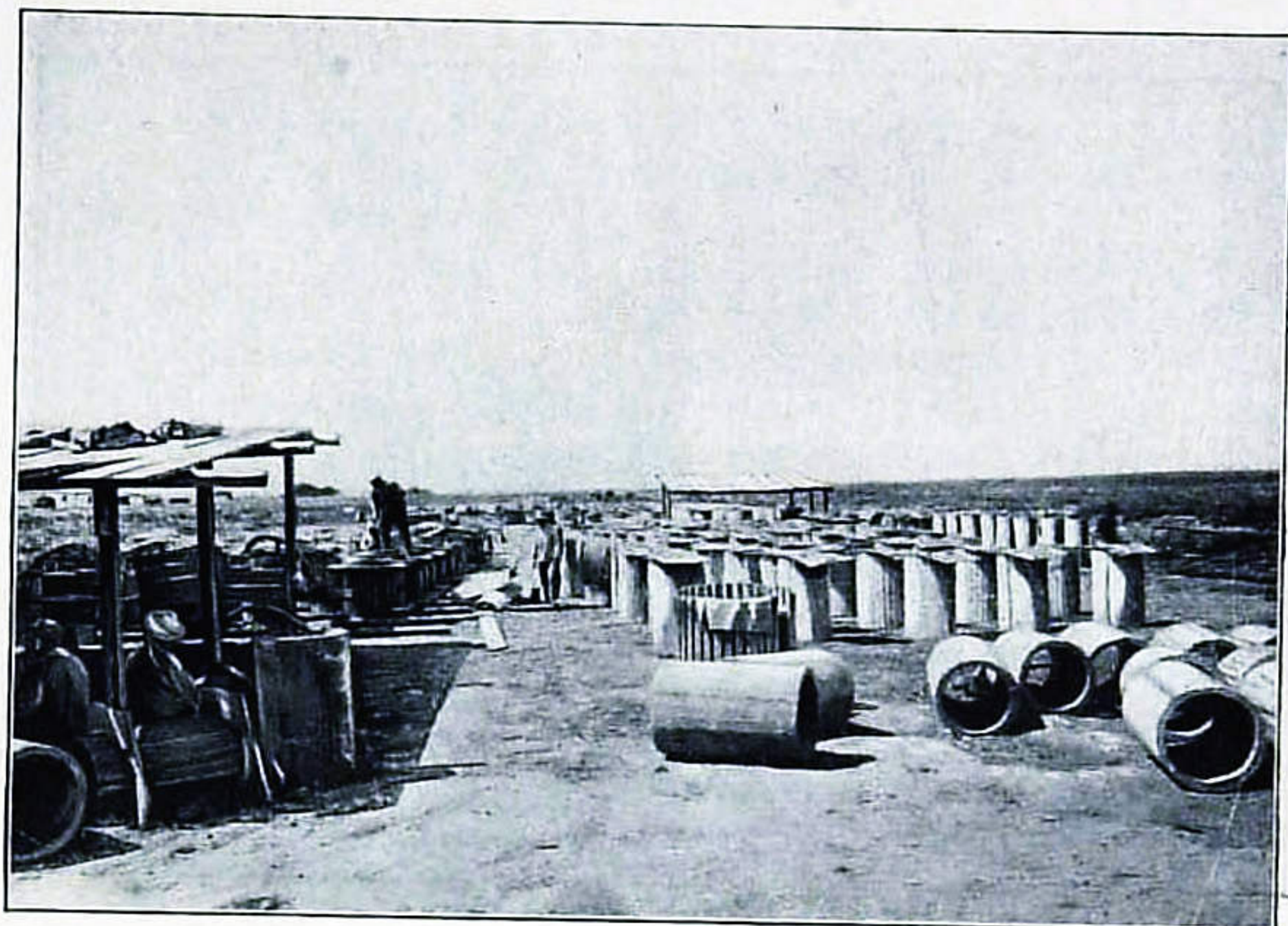
Заводская заготовка желѣзо-бетонныхъ трубъ при разъѣздѣ „Золотая Орда“ Ср. Азіатск. ж. д.
