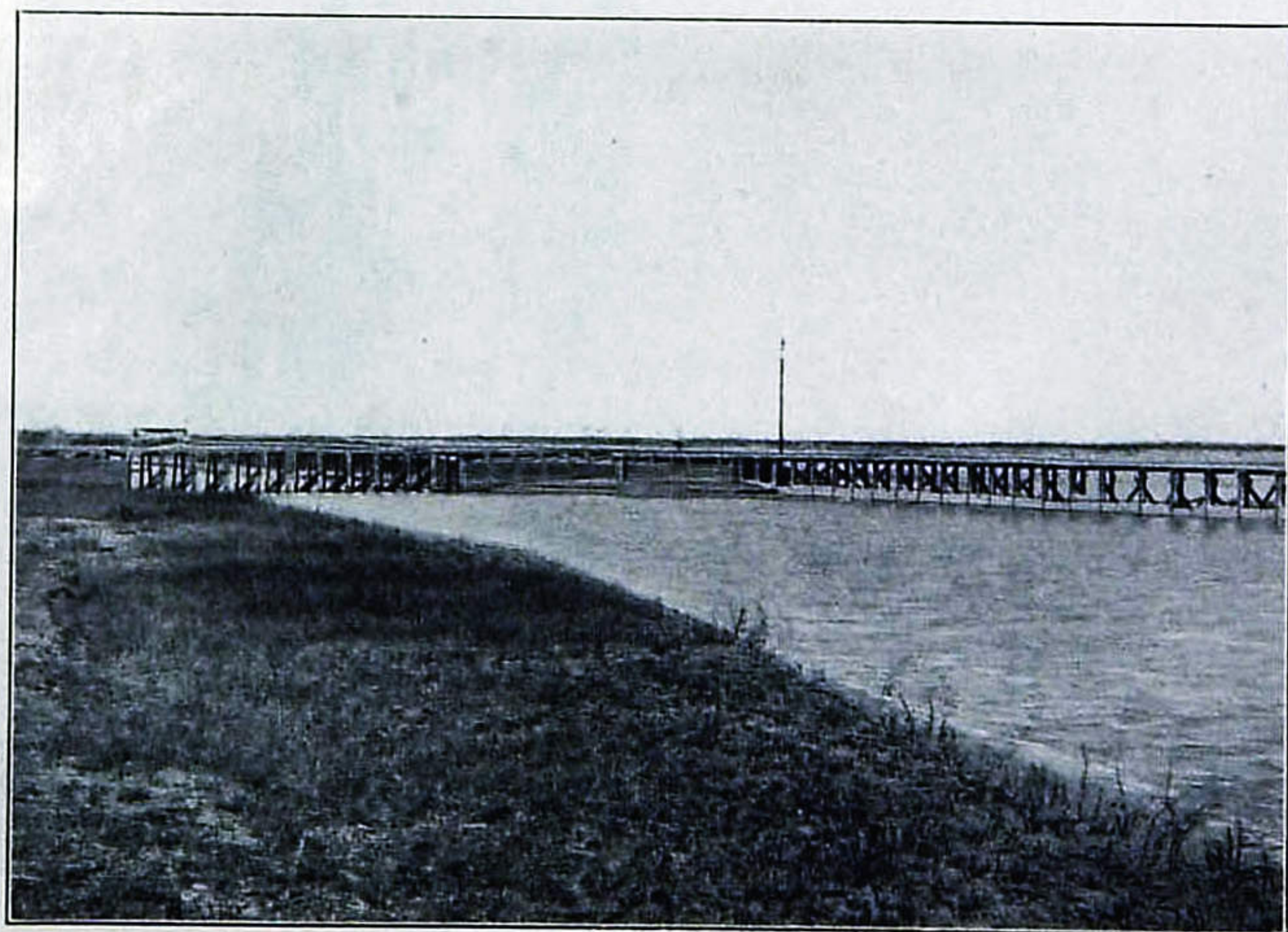
Косаральская плотина въ головѣ канала Николая I. Построена въ 1911 г.
