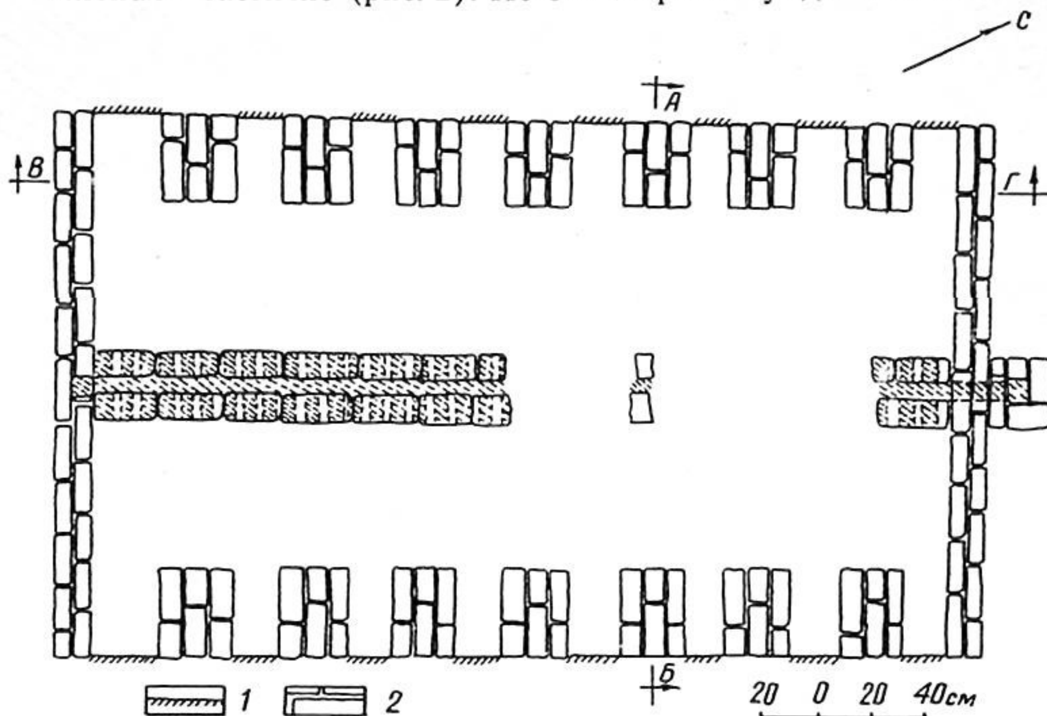
Рис. 1. План печи.
