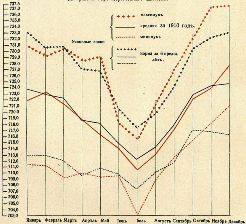
Диаграмма барометрическаго давления
