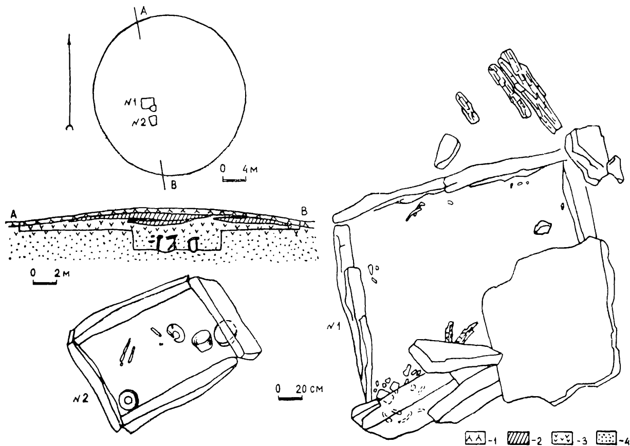
Рис. 2. Кургan 15. Условные обозначения: 1 — гумусный слой; 2 — глина темная, рыхлая; 3 — су- хоесть коричневатого-серая, плотная; 4 — плотный тонкозернистый песок с примесью гравия.
