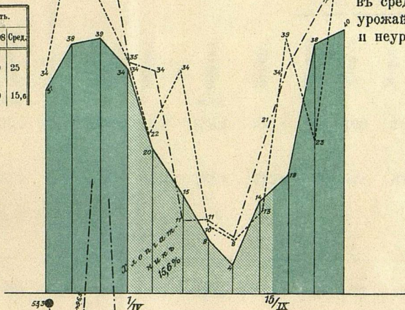
III. Диаграмма осадковъ: въ средній (закрашено), урожайный (1909), . . . . . и неурожайный (1908) годы. . . . .
