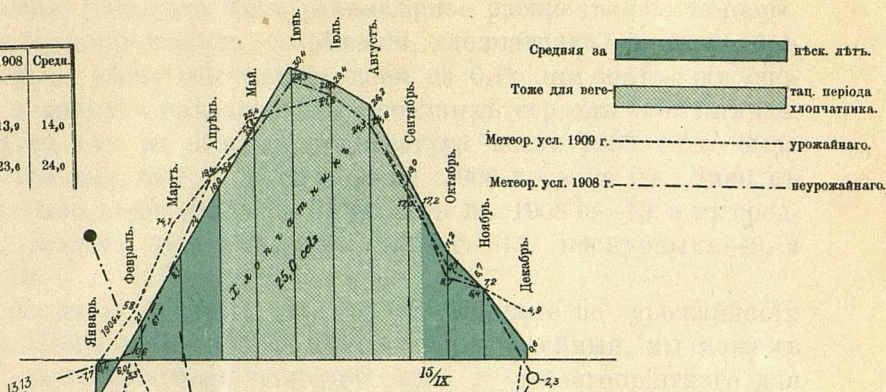
II. Диаграмма облачности: въ средній (закрашено), урожайный (1909), . . . . . и неурожайный (1908) годы. . . . .
