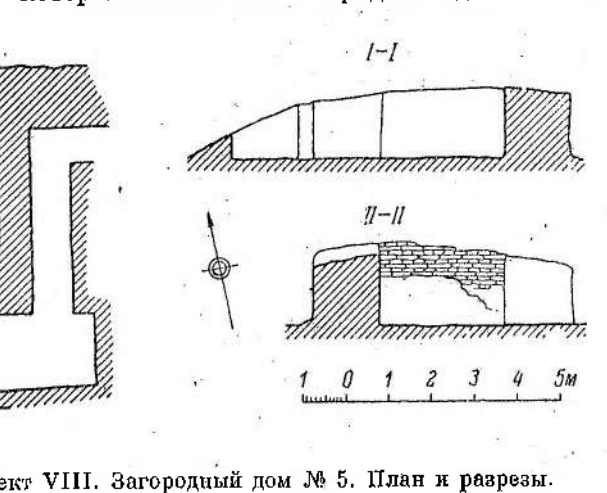
Рис. 13. Объект VIII. Загородный дом № 5. План и разрез.
