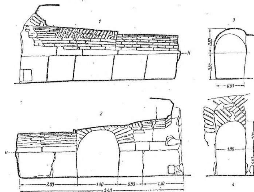
Рис. 16. Объект VIII. Загородный дом № 9. Свод коридора. 1, 2, — разрез свода коридора; 3 — пята свода; 4 — арка коридора.
