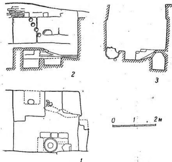
Рис. 12. Объект III. Восточная часть мастерской. 1 — план; 2 — разрез В-В; 3 — разрез С-С.
