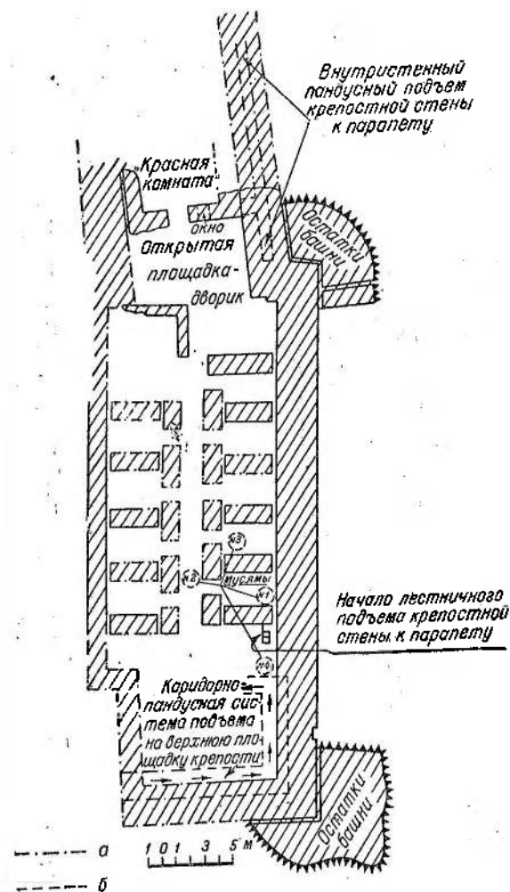
Рис. 20. Калаи-Боло. План верхней площадки в XI—XII вв. (первый этап третьего периода). а — реконструкция; б — стены, лежащие выше или ниже основного уровня площадки.
