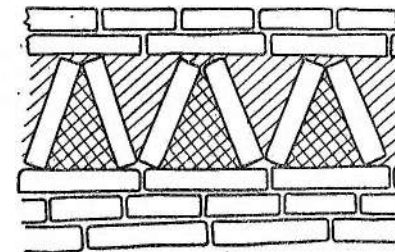
Рис. 11. Калай-Боло. Один из видов кирпичной кладки.
