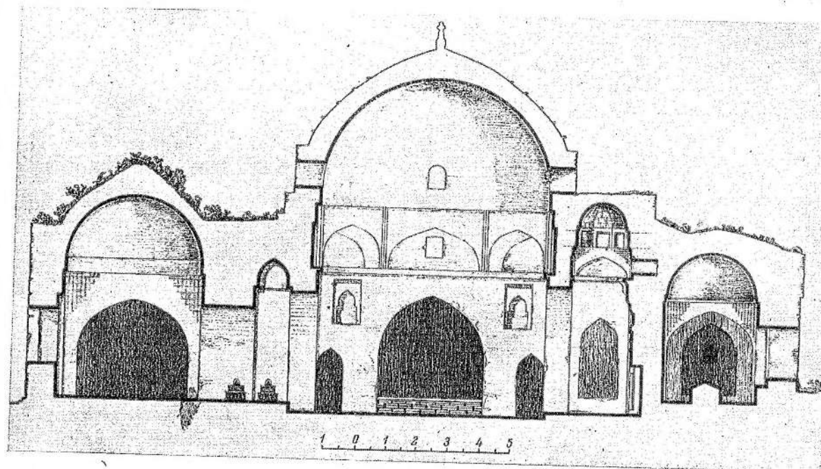
Рис. 6. Мавзолей Мухаммада Боишаро. Продольный разрез.
