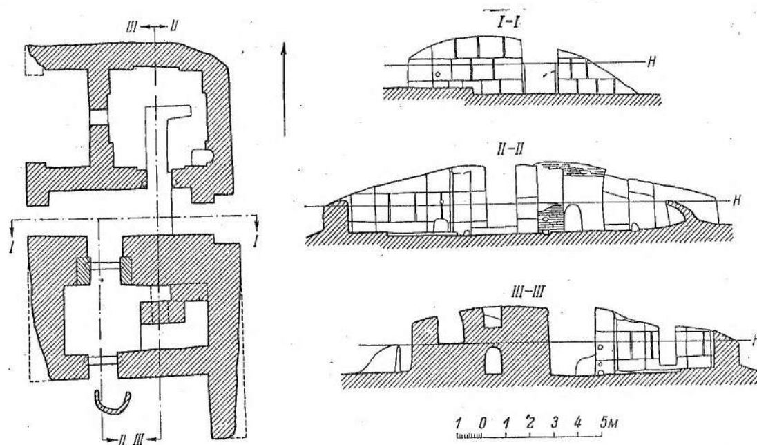
Рис. 9. Объект VIII. Загородный дом № 4. План и разрезы.
