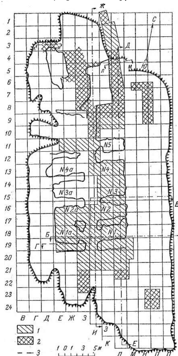
Рис. 3. Калаи-Боло. План с обозначением площадки раскопов и зачисток.
