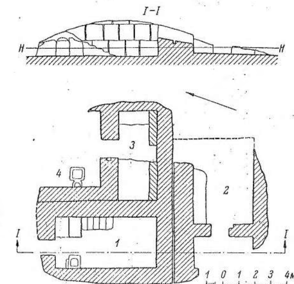
Рис. 10. Объект VIII. Загородный дом № 2. План и разрезы.
