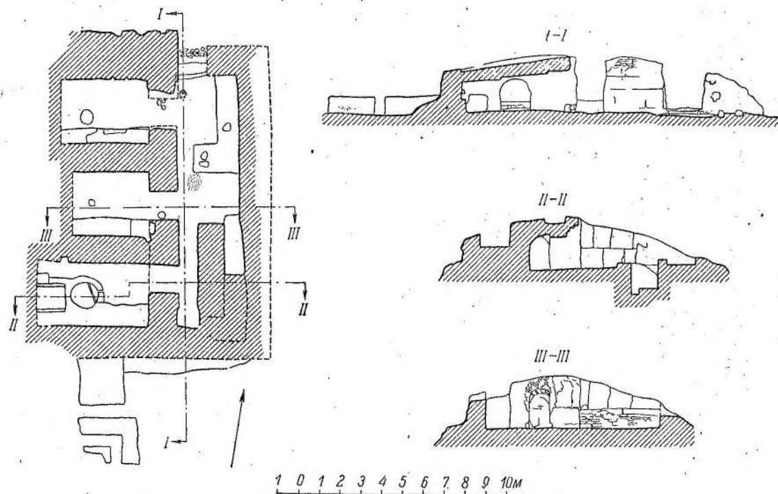
Рис. 14. Объект VIII. Загородный дом № 9. План и разрезы.
