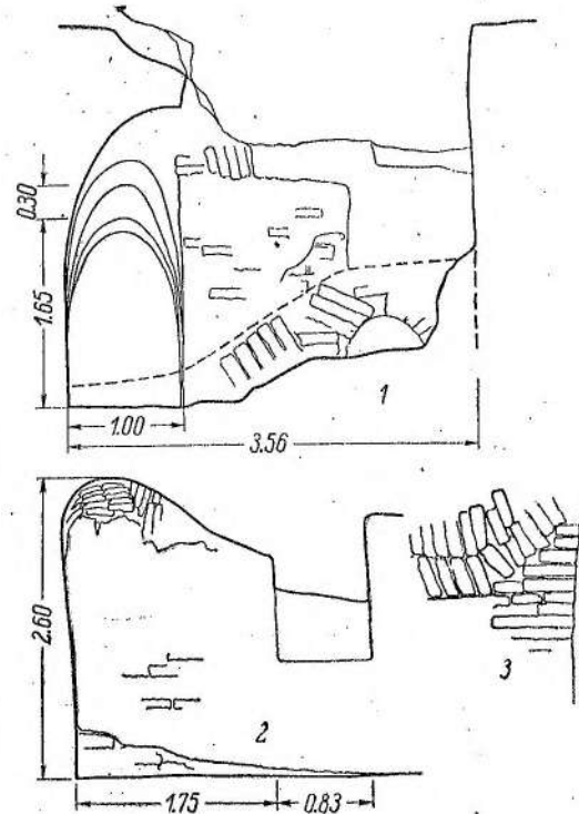
Рис. 18. Объект IX. Свод пандуса.
