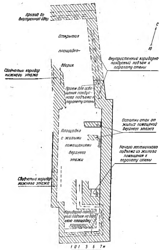
Рис. 7. Калаи-Боло. План верхней площадки (первый этап второго периода).
