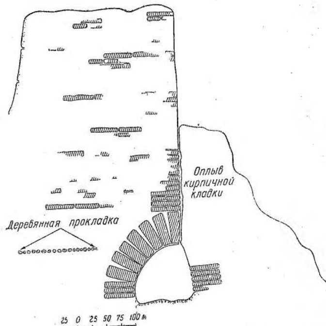
Рис. 9. Калай-Боло. Разрез Ж—З (по рис. 3) юго-восточного коридора восточной крепостной стены второго периода.
