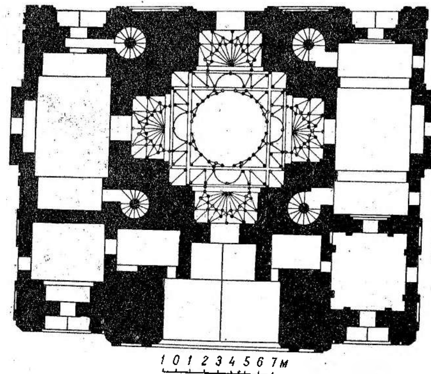
Рис. 17. Самарканд. Ишрат-Хона. План.
