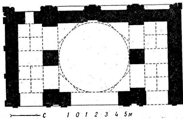
Рис. 13. Мавзолей Талхатан-Баба. План.
