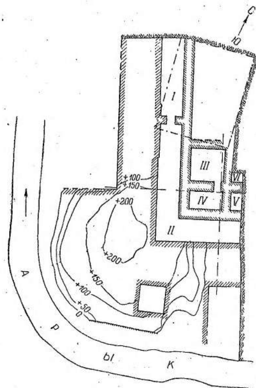
Рис. 5. Кей-Кобад-Шах. План раскопа 1953 г.
