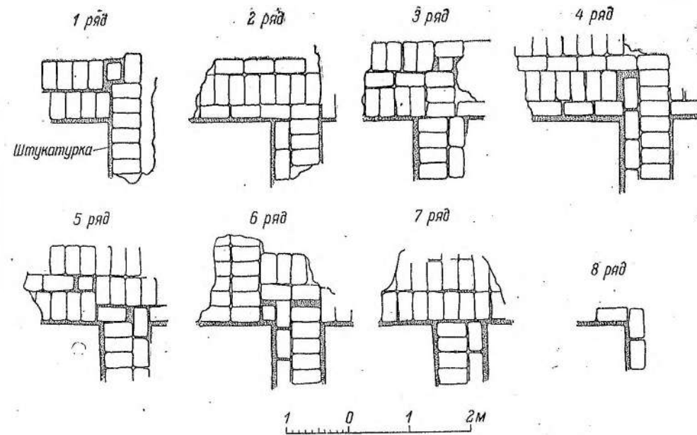
Рис. 15. Объект VIII. Загородный дом № 5. Перевязка сырцовый кладки.
