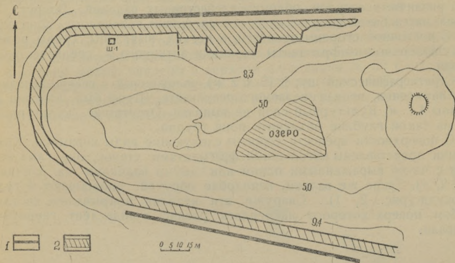
Рис. 1. План городища Каладжика: 1—стены античного периода, 2—стены средневекового периода.
