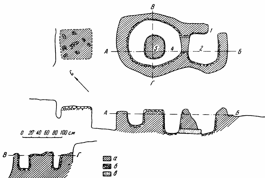
Рис. 2. Ер-Курган. Гончарная печь, план и разрезы печи. 1—устье топки; 2—топка; 3—жаропроводное отверстие; 4—обжигательная камера; 5—опорный столб; а—стены печи; б—ошлакованные поверхности; в—зола
