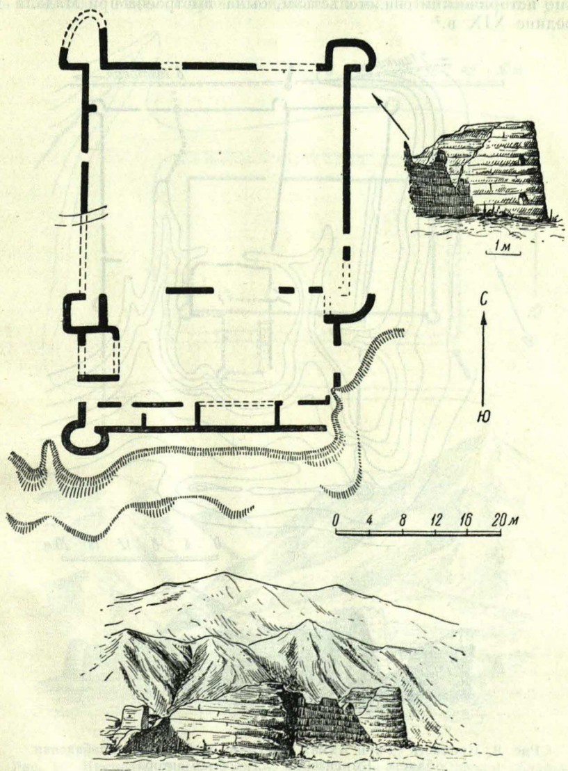
Рис. 8. Крепость Чолок-курган, Нарынская долина Киргизской ССР, вид с юго-востока (обмер автора).
