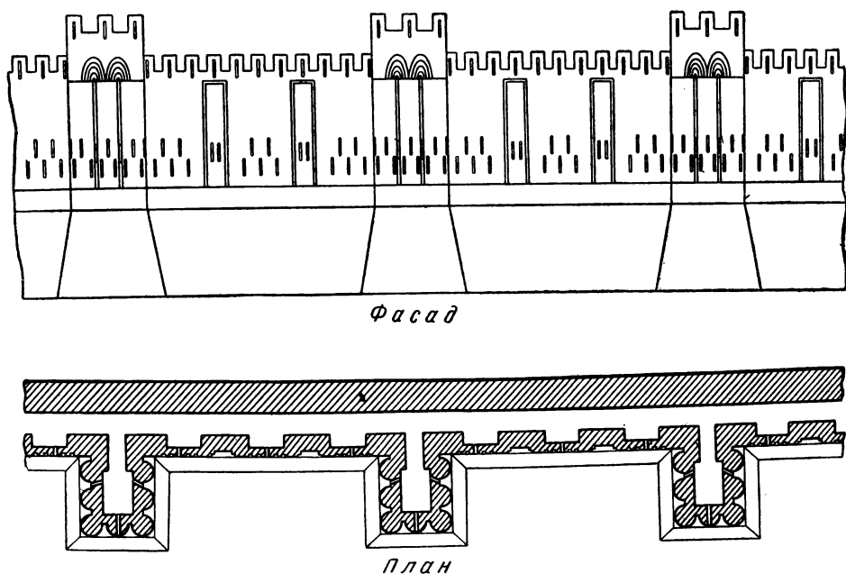
Рис. 6. Парфянская крепость «Чильбурдж» (чертежи реконструкции стен)
