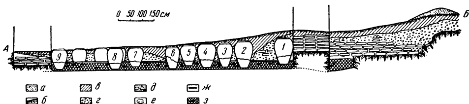
Рис. 18. Старая Ниса. Разрез хуманы I и хуманы II с обозначением мест находок парфянских документов. Условные обозначения: а — отвал земли 1936 г.; б — дермовой слой; в — натежно-надувной слой; г — разрушенная кирпичная кладка; д — сырцовые кирпичи; е — позднейшие погребения; ж — уровень пола; з — насыпной слой под полом со включениями остраконов
